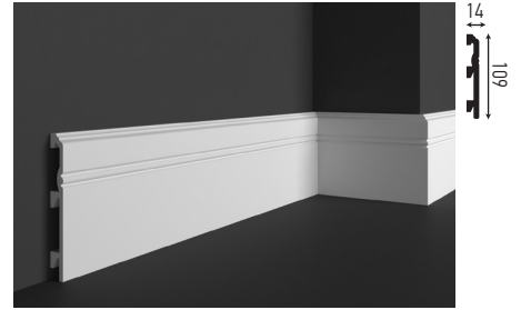
HCR 512 (F) 109 x 14 mm
