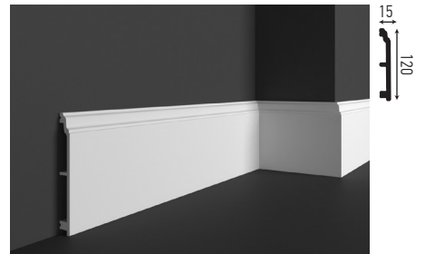
HCR 521 120 x 15 mm
