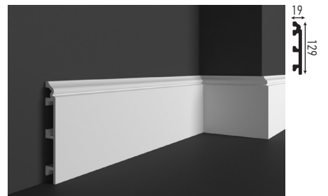
HCR 509 (F) 129 x 19 mm
