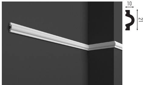
HCR 528 (F) 21 x 10 mm
